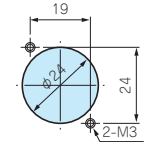
ノットリックコネクタ用 取付穴
