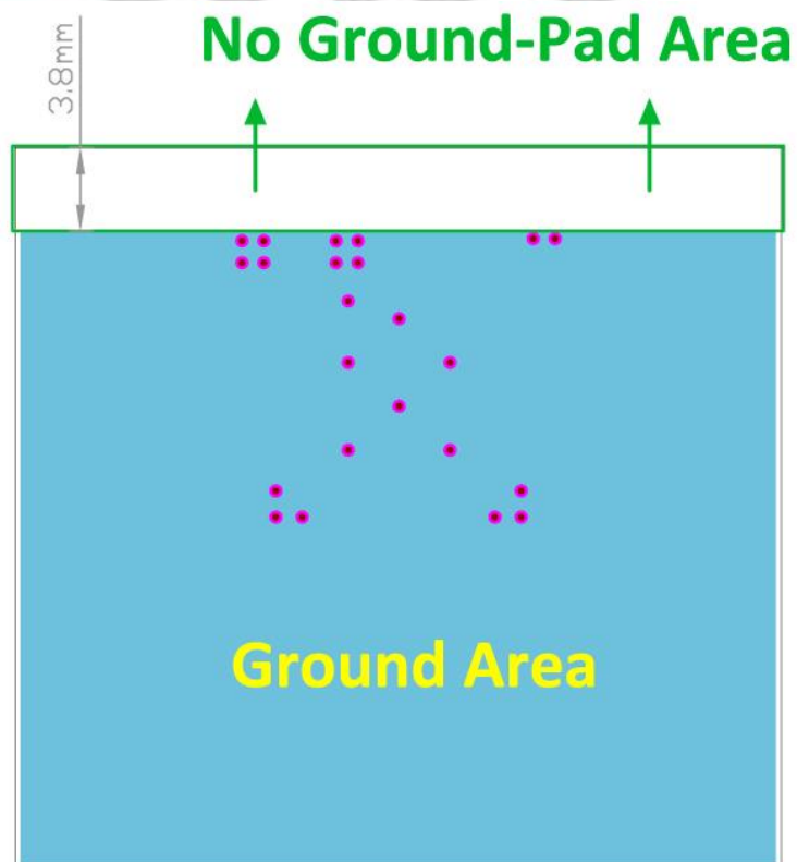
Bottom layer
