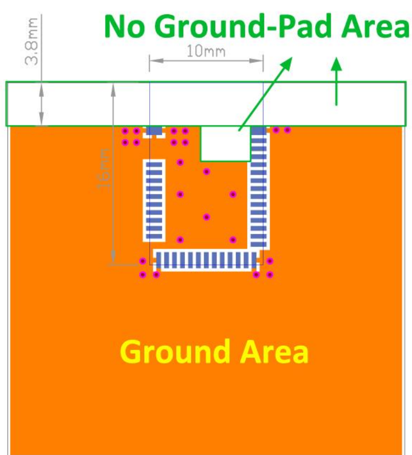
Top layer
