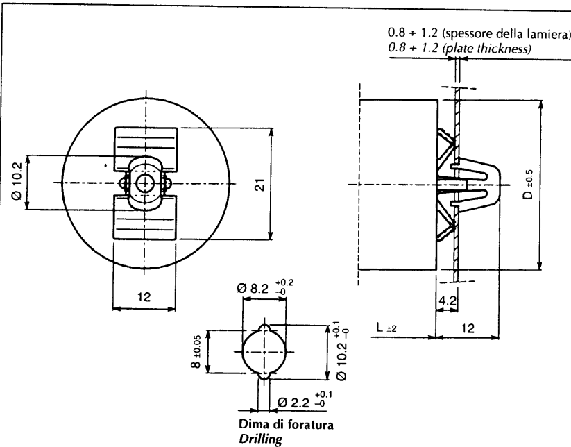
Fig. 6 Fissaggio rapido solo per dia 28, 32, 36, 40.
