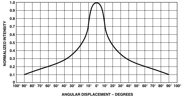
Figure 9. HLMP-Q102/-Q152
