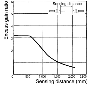
E32-T11L + E39-F3
