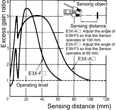
E32-T11L + E39-F3
