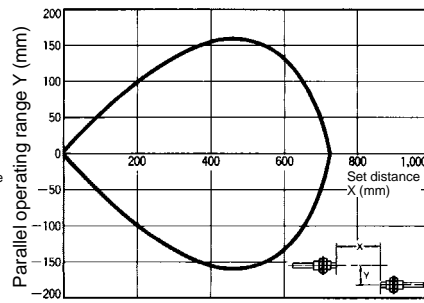
E32-T11
