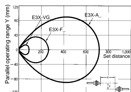
E32-T11L/T12L
