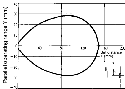
E32-T24
