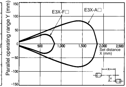
E32-T14
