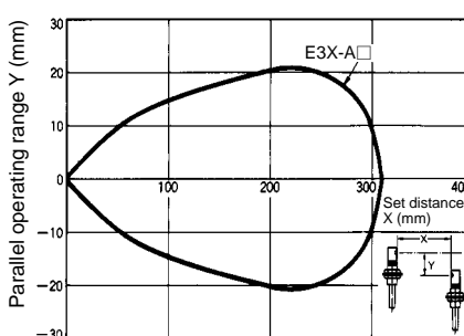
E32-TC200 + E39-F2
