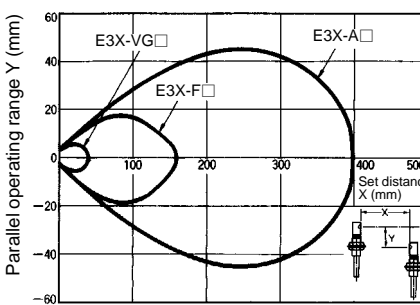
E32-T11L + E39-F2
