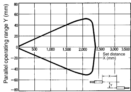
E32-T22S
