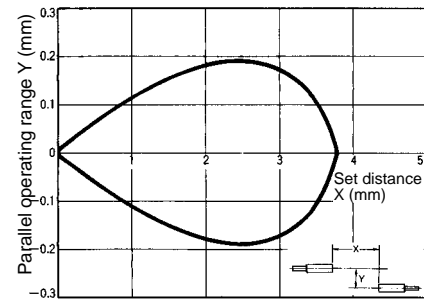
E32-T12F
