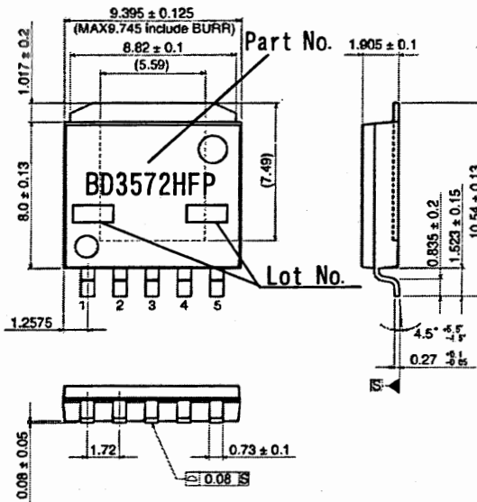
HRP-5 (Unit : mm)
