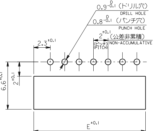
基板取付穴推奨寸法 (マウント面) RECOMMENDED P.C.B. BOARD HOLE DIMENSION (MOUNTING SIDE)
