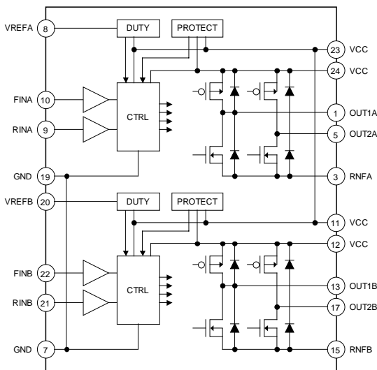
Fig. 31 BD6215FV
