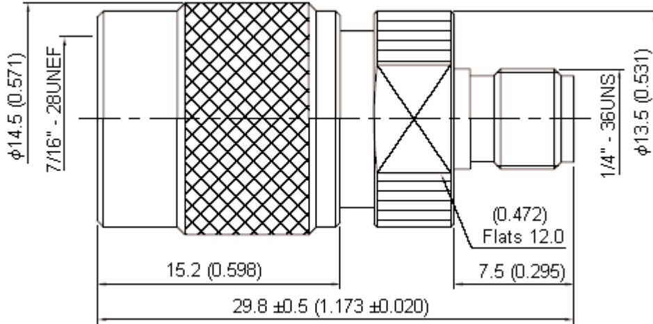
Dimensions : Millimetres (Inches)
