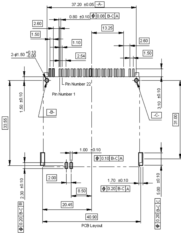
Dimensions : Millimetres
