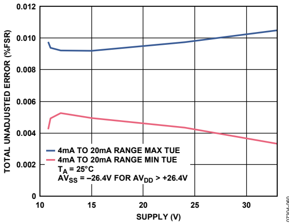
Figure 44. Total Unadjusted Error vs. AV DD , External R SET
