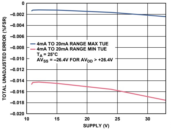
Figure 45. Total Unadjusted Error vs. AV DD , Internal R SET
