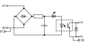
OB...IC 0100 24 V DC 24-48-60-115-230 V AC/DC
