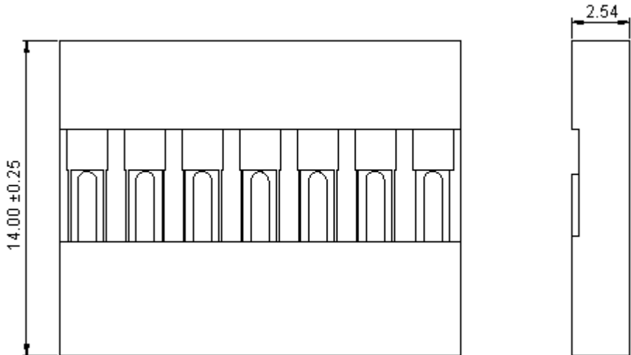
Dimensions : Millimetres
