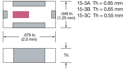
Case 15-3 (EIA 0805 / 2012)
