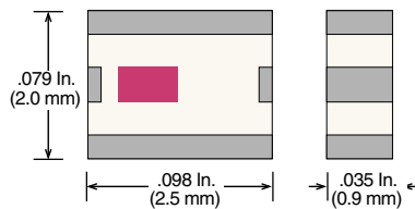
Case 39-1 (2025)
