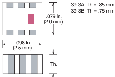
Case 39-3 (2025)
