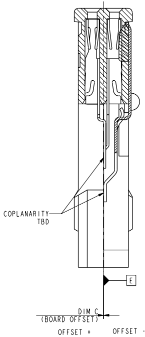
SECTION A-A SCALE 5.000
