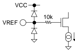
Fig.49 VREF
