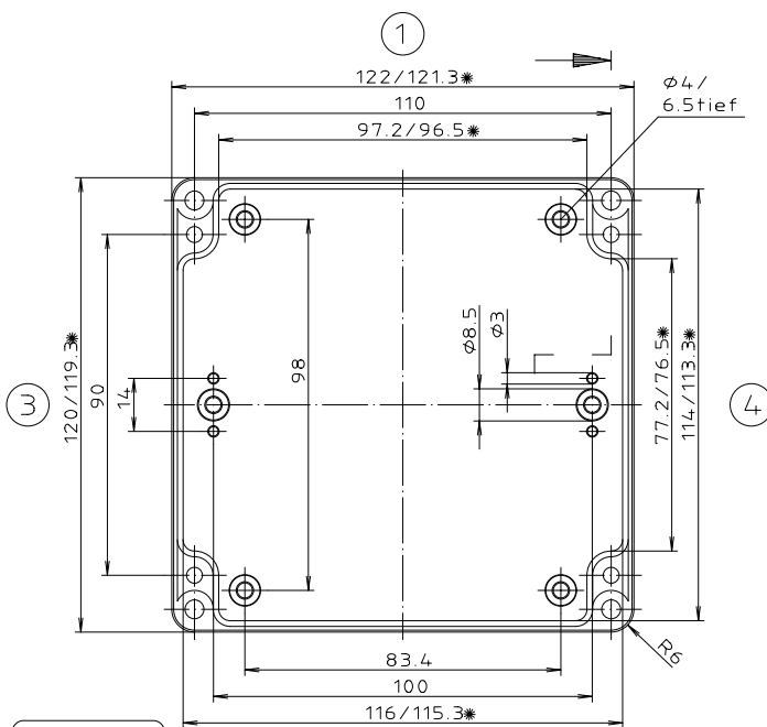
Unterteil
