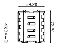
BOTTOM-PCB
