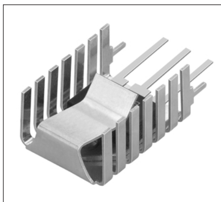
FK 243 MI 247 V 18,4 K/W mit Lötfahne für vertikalen Einbau
