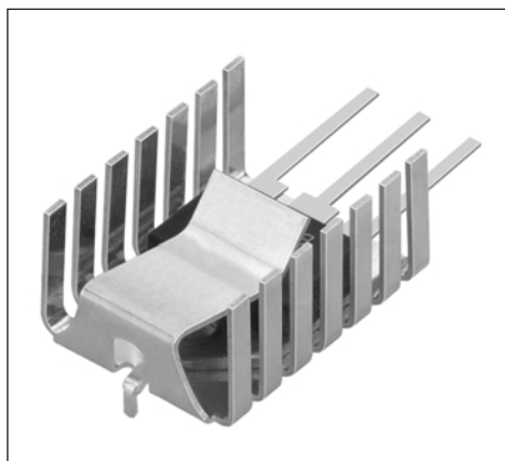
FK 243 MI 247 H 19 K/W mit Lötfahne für horizontalen Einbau
