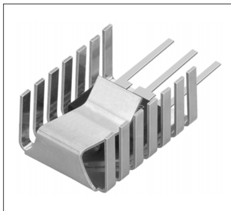
FK 243 MI 247 O 18,7 K/W ohne Lötfahne
