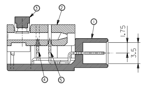
SECT A-A
