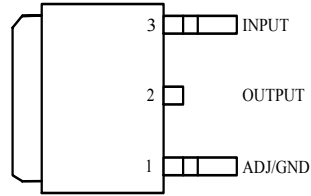
V2 Package (TO-252)
