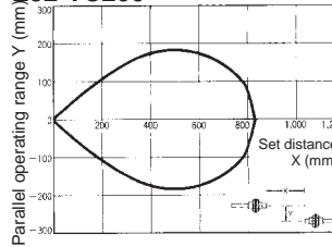
E32-T11L with E39-F2
