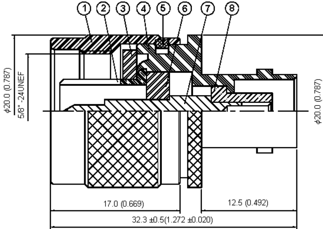
Dimensions : Millimetres (Inches)
