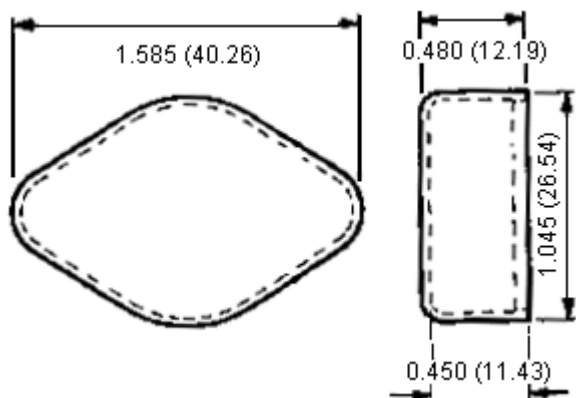
Dimensions : Inches (Millimetres)
