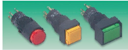
Round Bezel = 14 dia. Square Bezel = 14 14 Rectangular Bezel = 14 18
