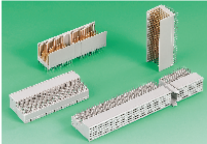
335-4763 335-4830 335-4568 335-4600
